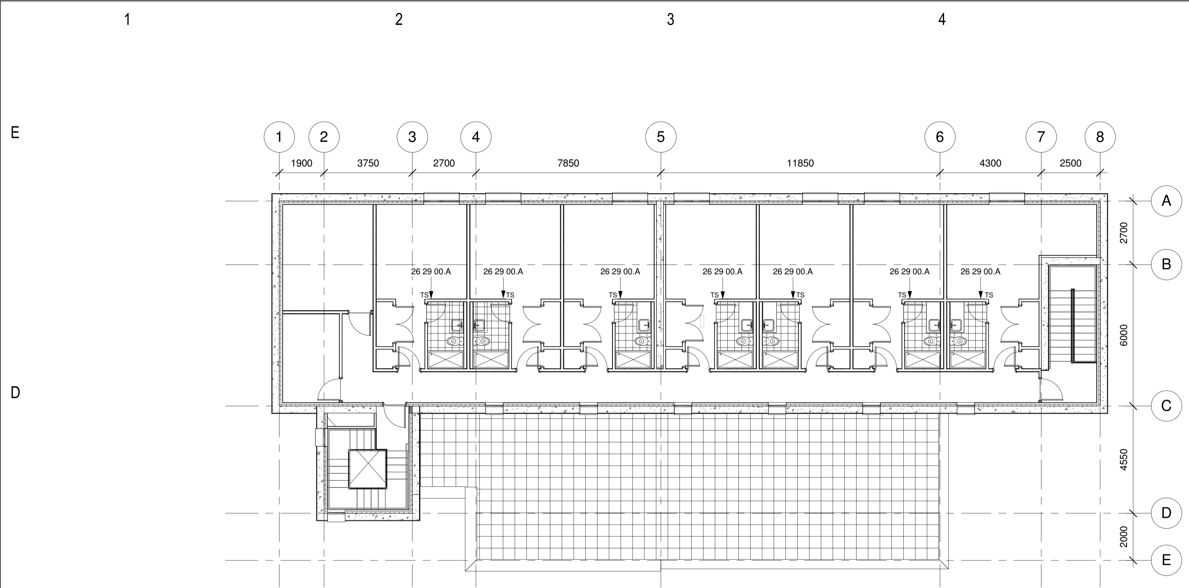
C1 Level 2 Floor Plan 1 : 100
